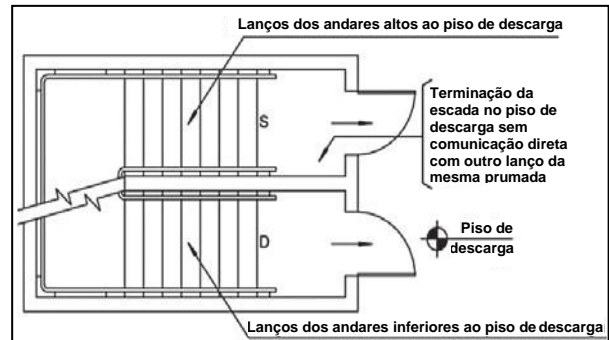
Figura 3 – Segmentação das escadas no piso da descarga
