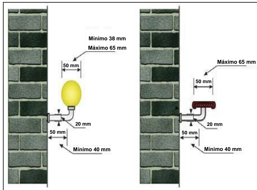
Figura 15 – Dimensões de guardas e corrimãos
