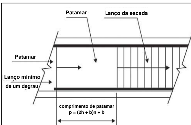
Figura 5 – Lança mínimo e comprimento de patamar
