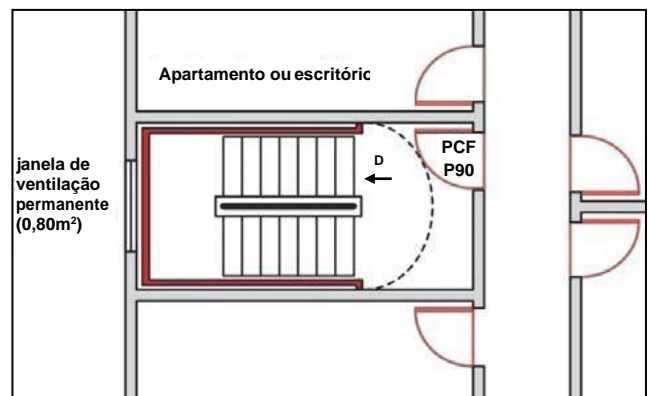
Figura 7 – Escada enclausurada protegida
