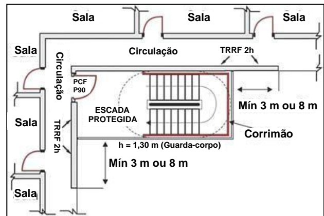
Figura 13 – Escada aberta externa
