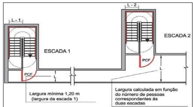
Figura 17 – Dimensionamento de corredores de descarga
