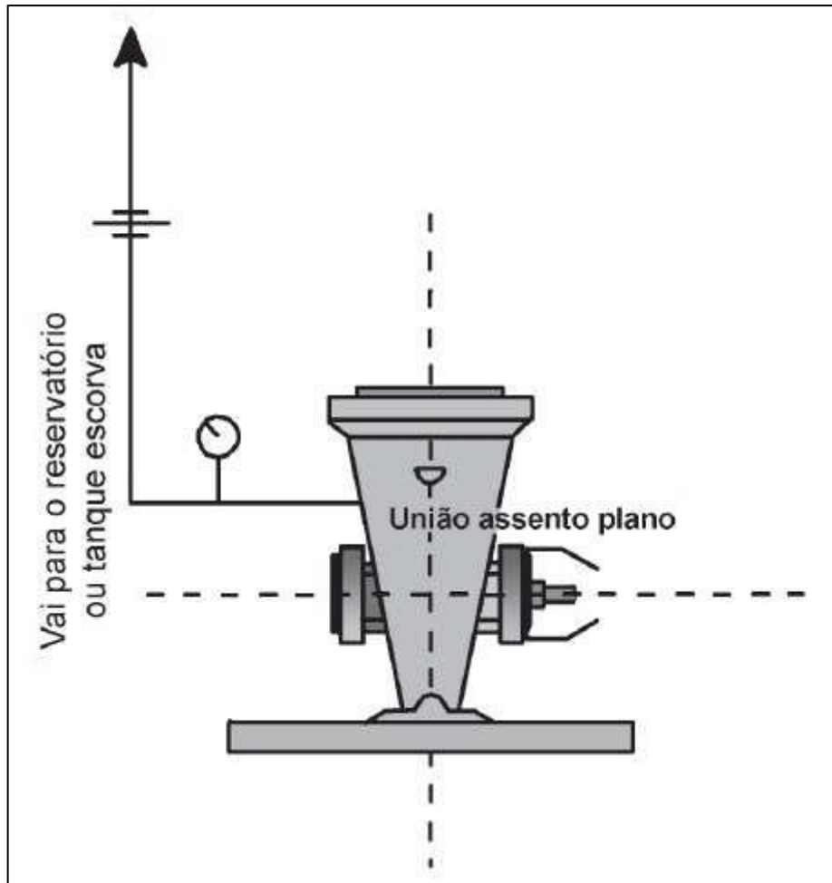
Figura C.7 – Arrefecimento da bomba principal elétrica
