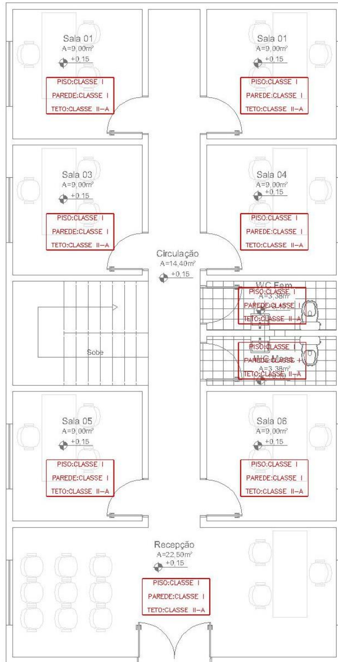
Planta Baixa Térreo Esc. 1/50
