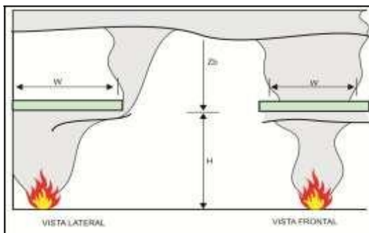
Figura 41 – Coluna de fumaça saindo de um balcão
