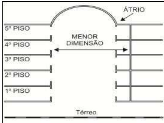
Figura 33 – Átrio considerado aberto de um lado e fechado do outro
