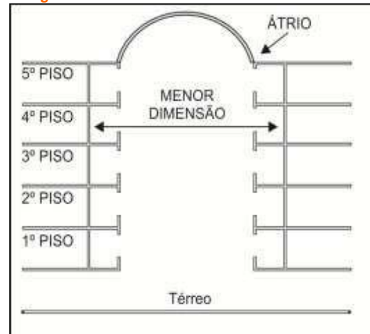
Figura 32 – Modelo 2 de átrios cobertos fechados
