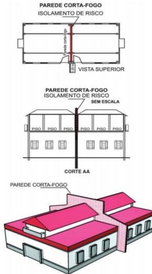
Figura 15 - Isolamento obtido por parede corta-fogo
