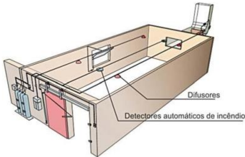
Figura 50 - Sistema de CO 2
