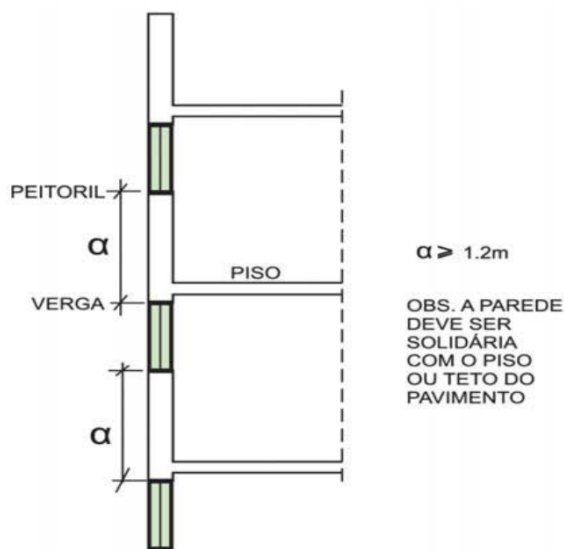
Figura 17 - Distância de afastamento entre verga e peitoril
