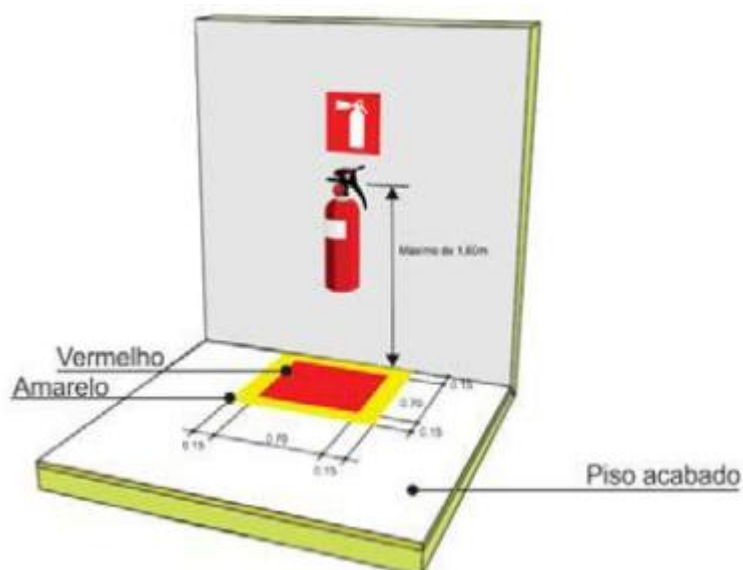
Figura 37 - Detalhe de instalação de extintores em áreas sujeitas à obstrução
