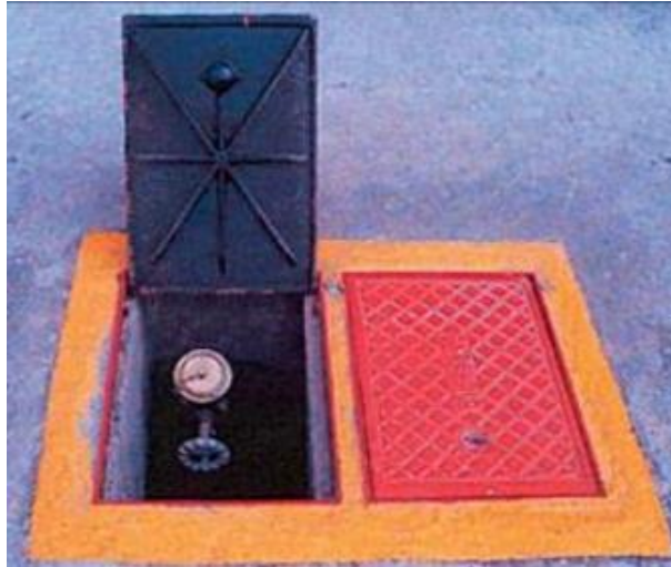
Figura 39 - Registro de recalque para bombeiros
