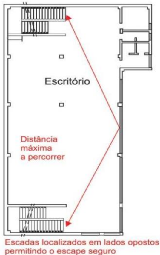
Figura 24 - Localização e caminhamento para acesso a uma escada
