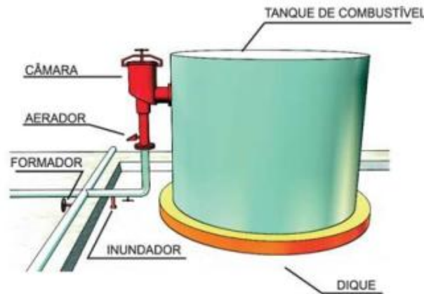
Figura 48 - Detalhe de câmara de espuma
