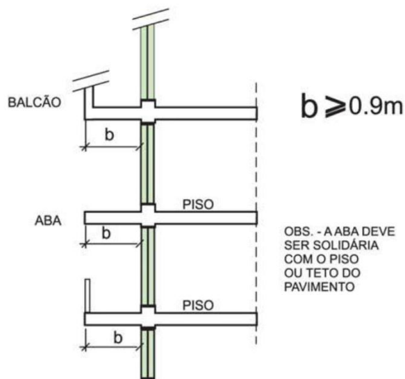
Figura 18 - Compartimentação por aba horizontal ou balcão
