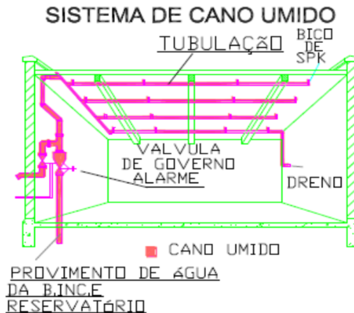
Figura 44 - Esquema de uma rede de chuveiro automático
