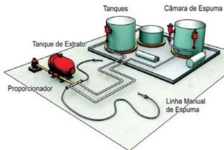
Figura 47 - Sistema semifixo
