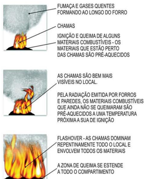
Figura 21 - Evolução da propagação nos materiais
