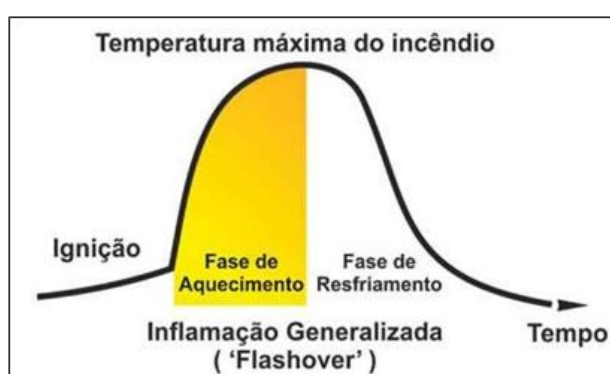
Figura 3 - Curva temperatura tempo de um incêndio
