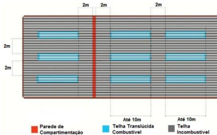
Figura 2 - Afastamento de telhas combustíveis translúcidas
