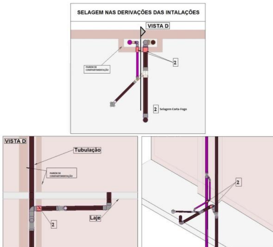
Figura D3 - Selagem nas derivações das instalações
