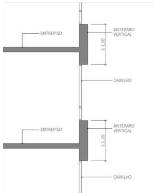
Figura C2 - Modelo de compartimentação com anteparo vertical
