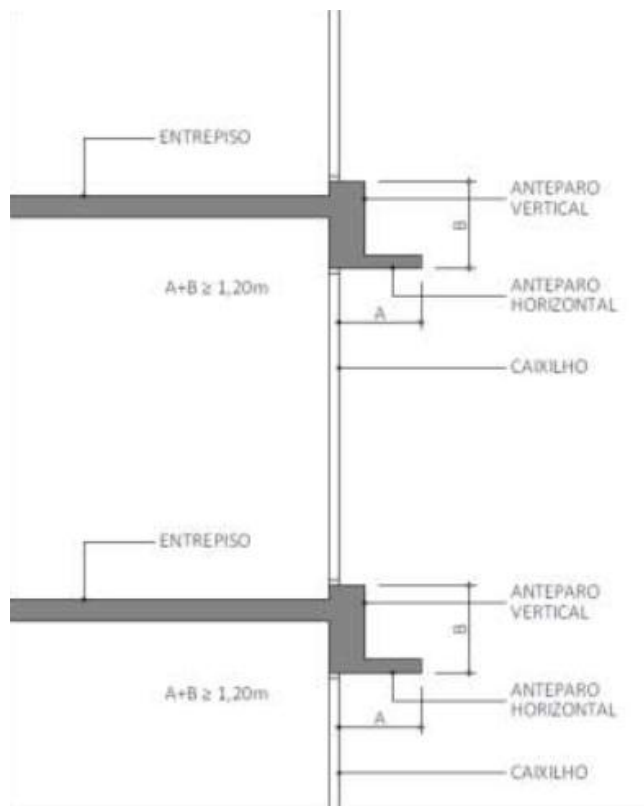
Figura C4 - Modelo de compartimentação com somatório de anteparos
