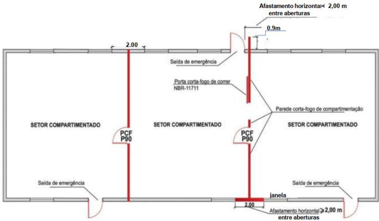
Figura C1 - Modelo de Compartimentação horizontal
