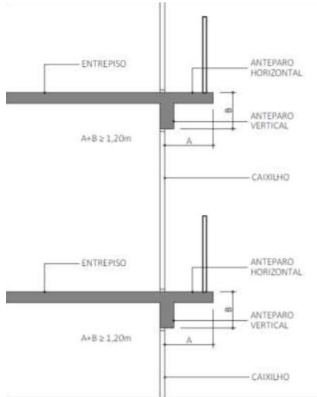
Figura C5 - Modelo de compartimentação com somatório de anteparos
