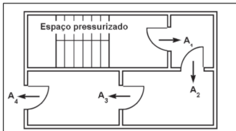
Figura 2 - Trajetórias de escape do ar em série
