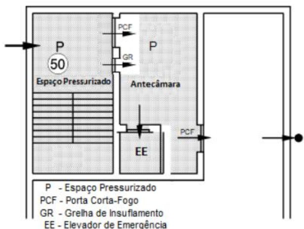
Figura 5 - Pressurização de antecâmara do elevador de emergência contígua a escada
