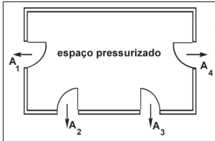
Figura 1 - Trajetórias de escape do ar em paralelo
