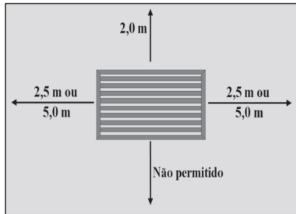
Figura 9 - Distâncias mínimas de aberturas à tomada de ar
