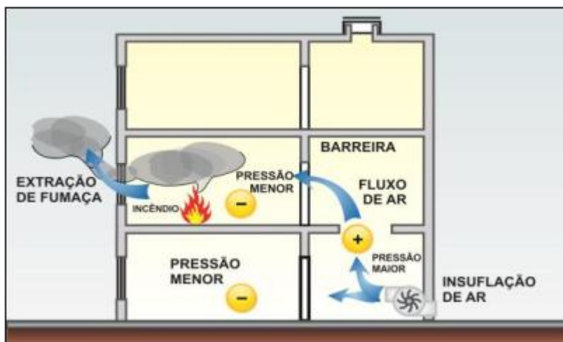
Figura 3 - Diferencial de pressão
