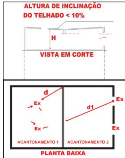
Figura 15 - Distâncias entre saídas de extração de fumaça
