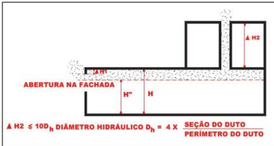
Figura 17 - Diâmetro hidráulico
