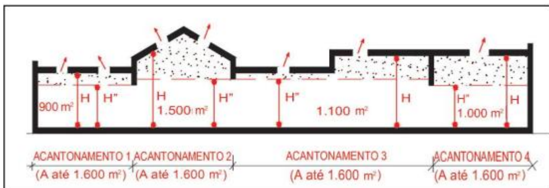
Figura 16 - Altura de referência diversificada por acantonamento
