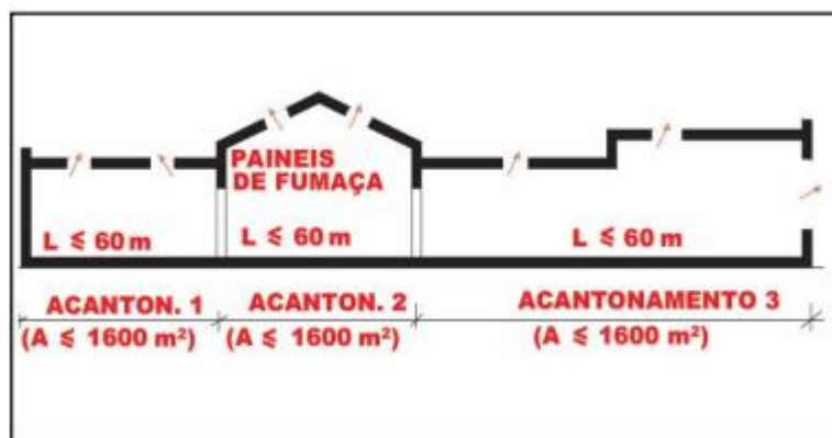
Figura 13 - Divisão em áreas de acantonamento
