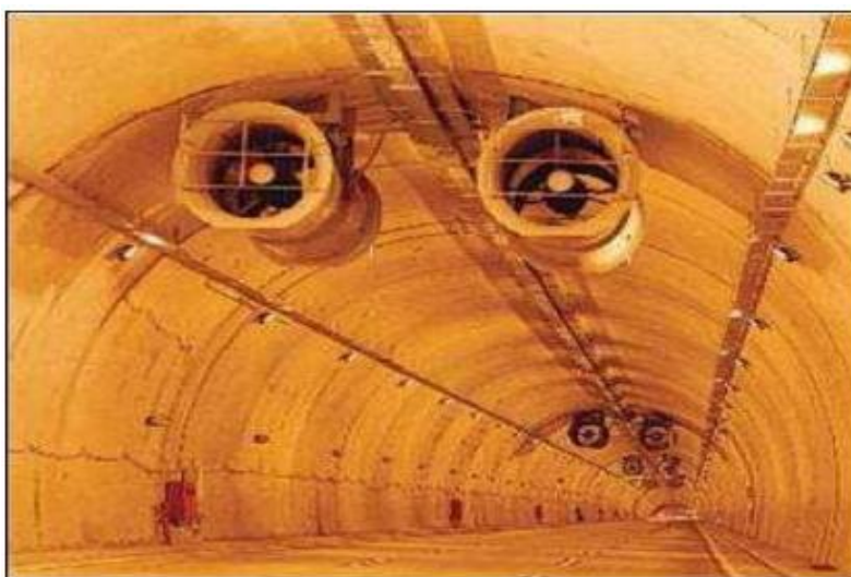
Figura 1 - Sistema de ventilação longitudinal
